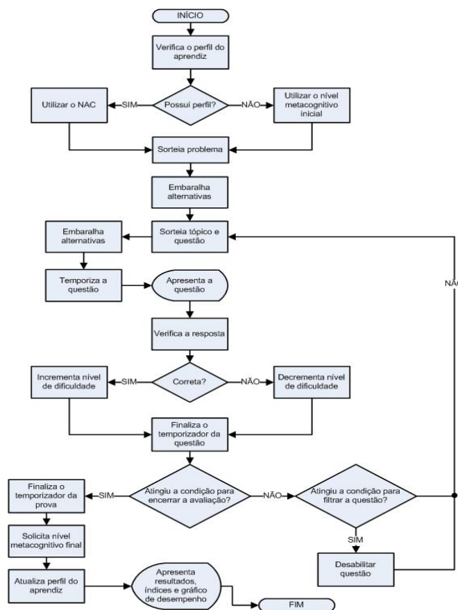
Figura 8. Fluxograma Simplificado do Algoritmo adaptativo
