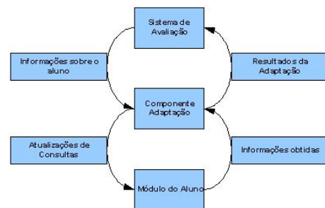
Figura 4. Estrutura genérica adaptada de Brusilovsky [16] e Henze [19].
